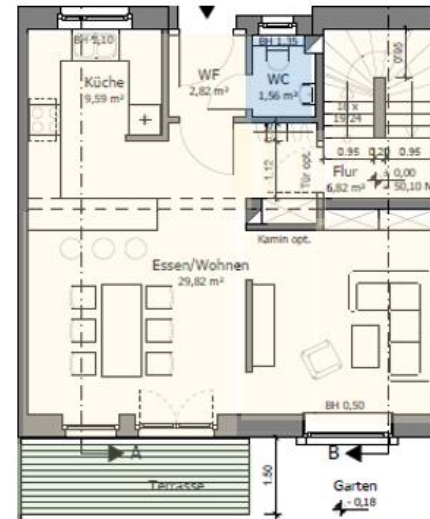
EG
